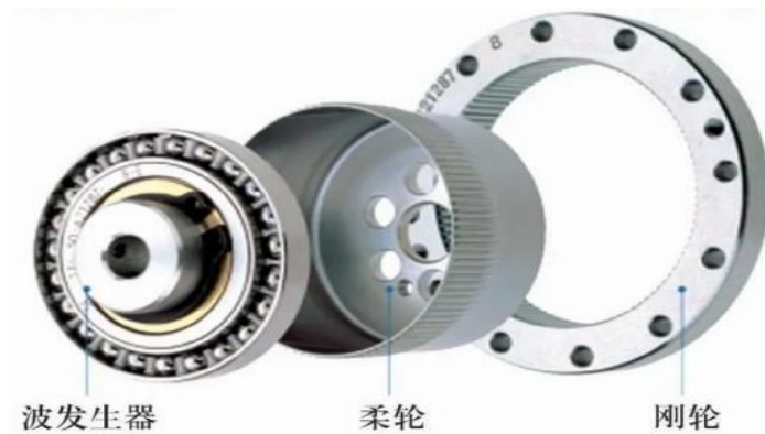
谐波减速机
