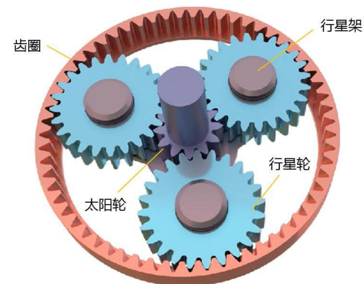
行星齿轮减速机
