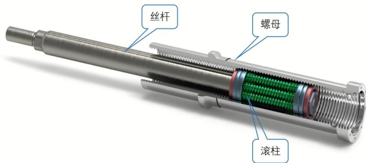
行星滚柱丝杠
