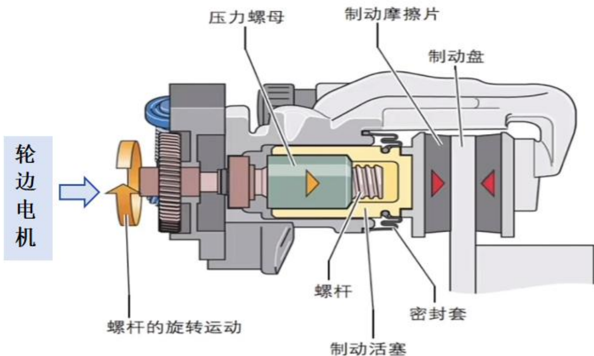
EMB结构图
